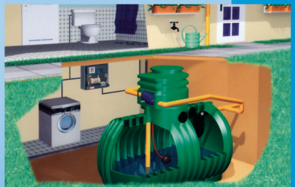
Regenwasser-Hausanlagen
